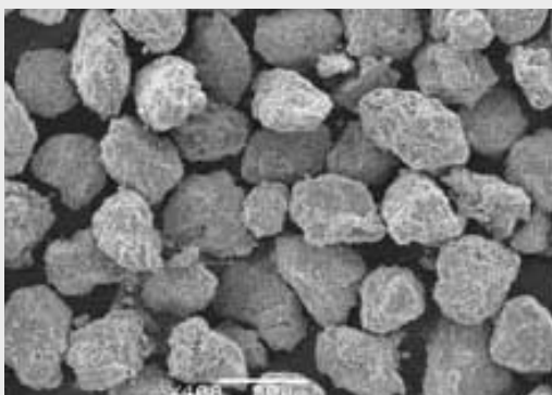
Απεικόνιση των κόκκων της νανοκρυσταλλικής σκόνης χρωμιομαγνησίου κάλυβα.
